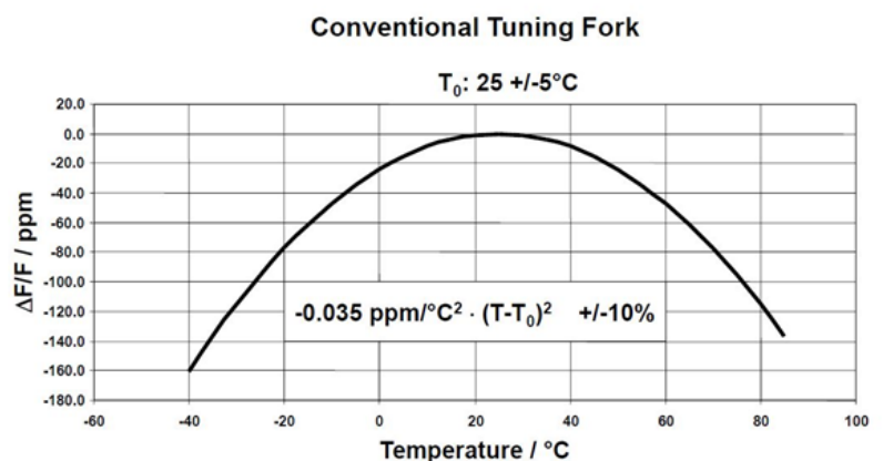
Bild 2: Der Temperaturgang (Frequenzabweichung über der Temperatur) eines Stimmgabelquarzes wird durch die Formel \text{Abweichung [ppm]} = -PC \text{ [ppm/}^\circ\text{C}^2] \cdot (T - T_0)^2 beschrieben, die im Koordinatensystem einer nach unten geöffnete Parabel mit Scheitelpunkt bei T_0 = +25 \text{ }^\circ\text{C} \pm 5 \text{ }^\circ\text{C} (Bezugstemperatur) entspricht.
